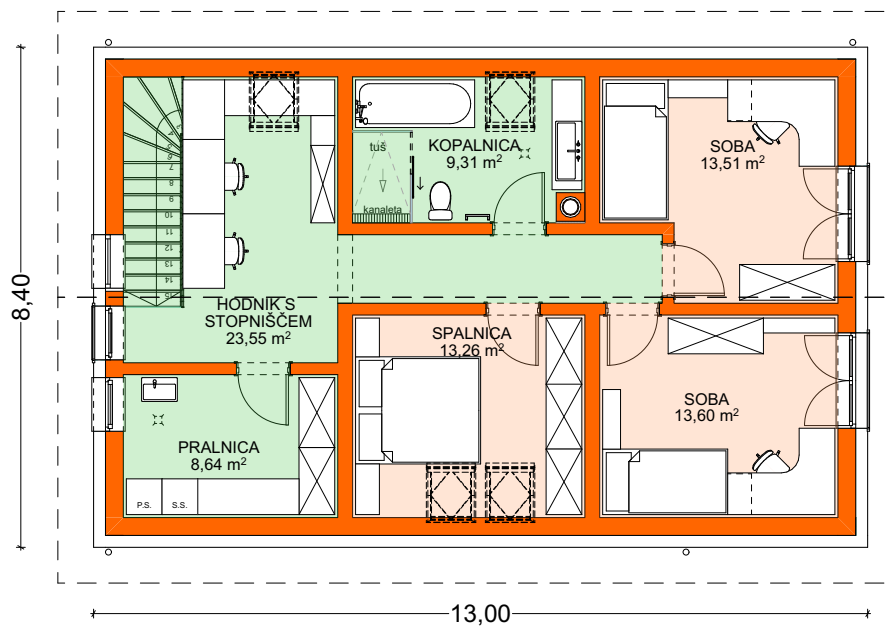
NADSTROPJE
