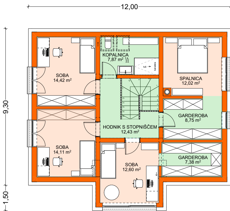
NADSTROPJE
