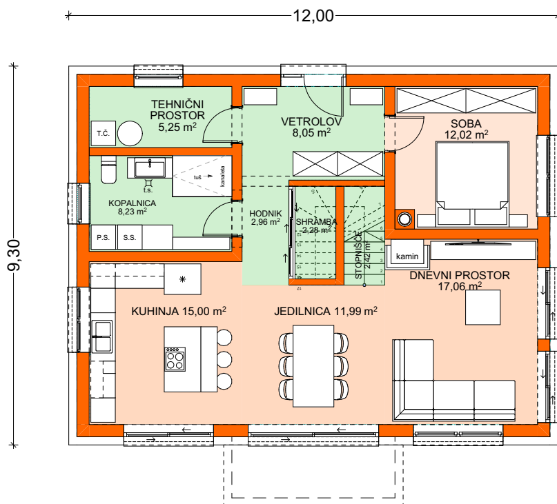
PRITLIČJE
