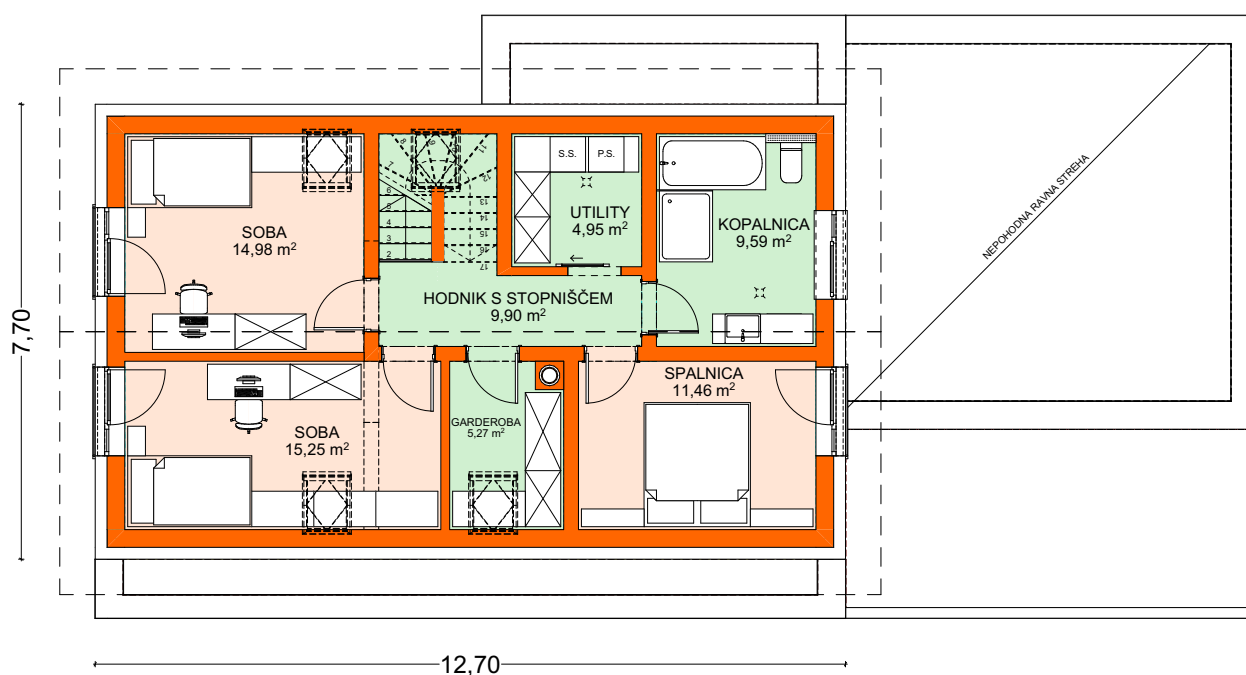
NADSTROPJE
