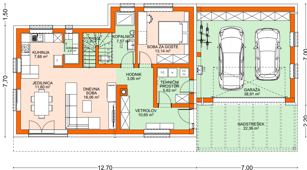
PRITLIČJE
