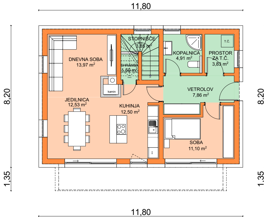
PRITLIČJE
